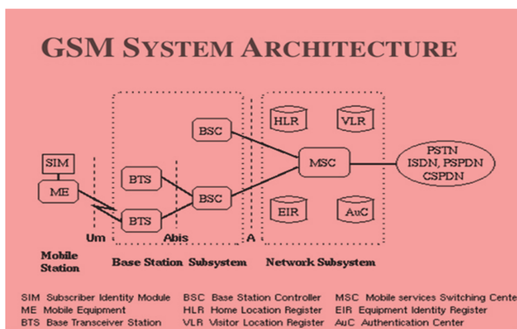
Fig. 3. GSM Architecture (Kurose, 2005)
